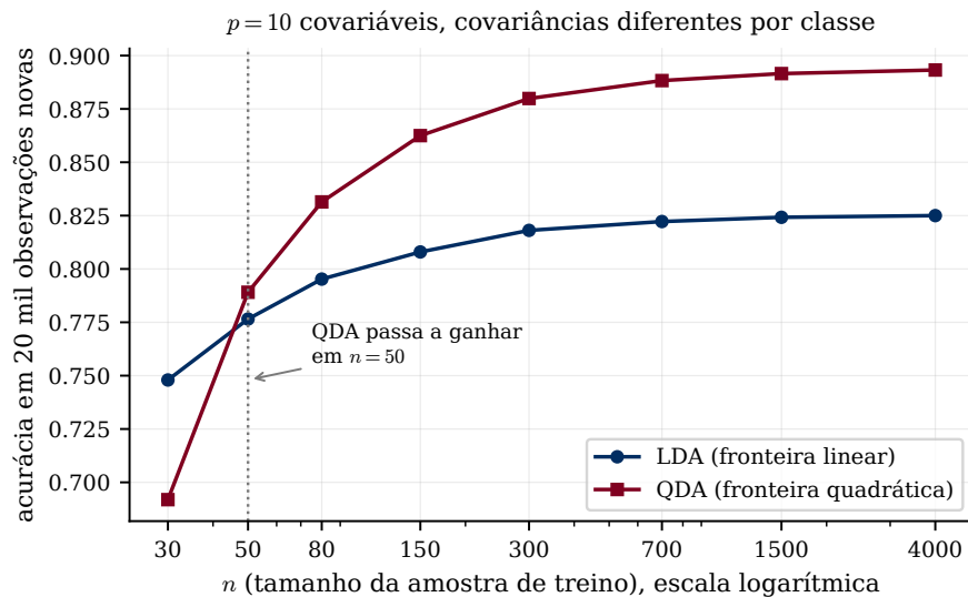
Figura 1: Acurácia dos dois métodos em função de n , com p = 10 covariáveis e covariâncias genuinamente diferentes por classe — ou seja, num cenário em que o QDA está certo e o LDA está errado . Ainda assim, com n = 30 o LDA ganha (0,748 contra 0,692): não há dados para estimar 110 parâmetros de covariância, e a variância do QDA supera o viés do LDA. A partir de n = 50 o jogo vira, e em n = 4000 o QDA abre sete pontos percentuais. Médias de 120 repetições, avaliadas em 20 000 observações novas.
