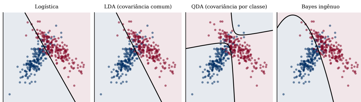
Figura 2: Fronteiras de decisão em duas classes gaussianas com covariâncias diferentes ( n = 400 ). Logística e LDA chegam a retas quase idênticas por caminhos completamente distintos — uma modelando \mathbb{P}(Y \mid \mathbf{x}) direto, a outra modelando f(\mathbf{x} \mid Y) e invertendo. O QDA, livre da hipótese de covariância comum, curva a fronteira e acompanha o formato de cada nuvem: é o modelo correto para estes dados. O Bayes ingênuo também curva, mas erra o ângulo: ele supõe as duas covariáveis independentes dentro de cada classe, e aqui elas não são.
